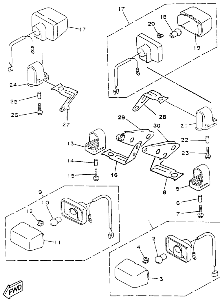
FIG. 37 - SINALIZADORES (PISCA-PISCA)
