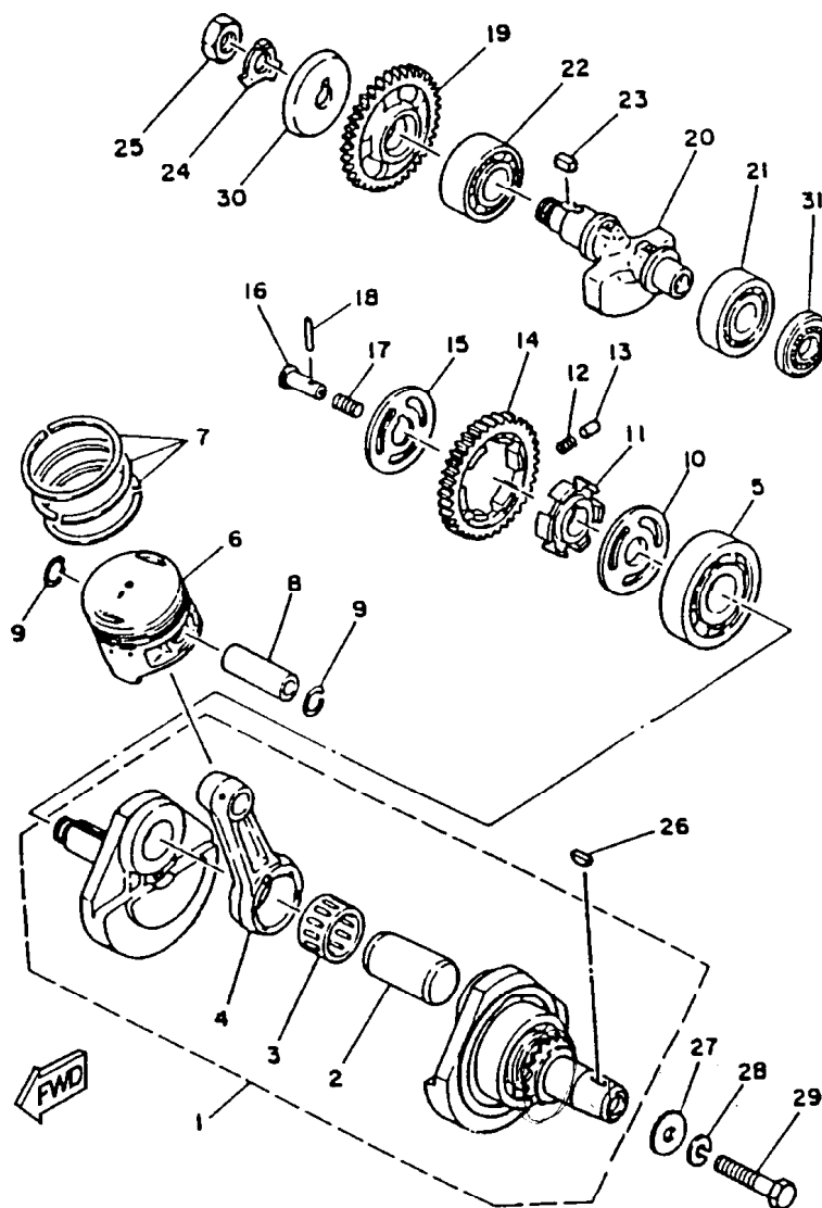
FIG. 03 - VIRABREQUIM E PISTÃO
