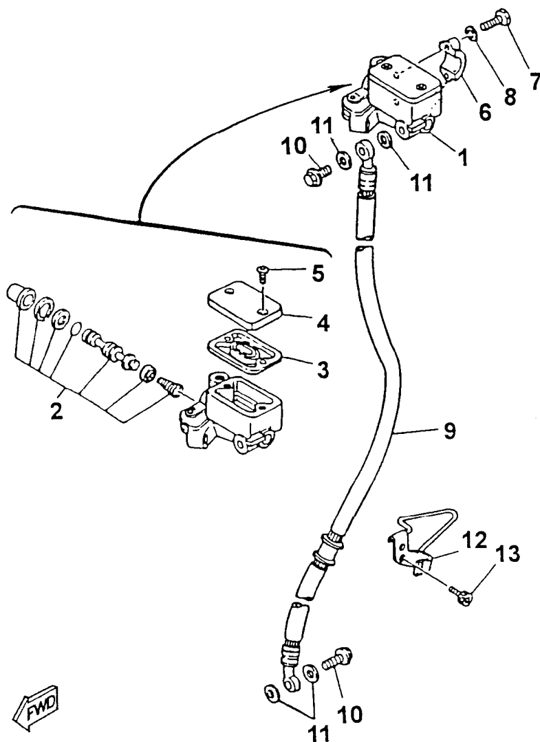
FIG. 33 - CILINDRO MESTRE
