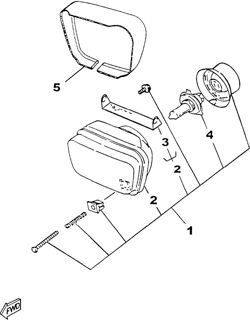
FIG. 32 - FAROL DIANTEIRO
