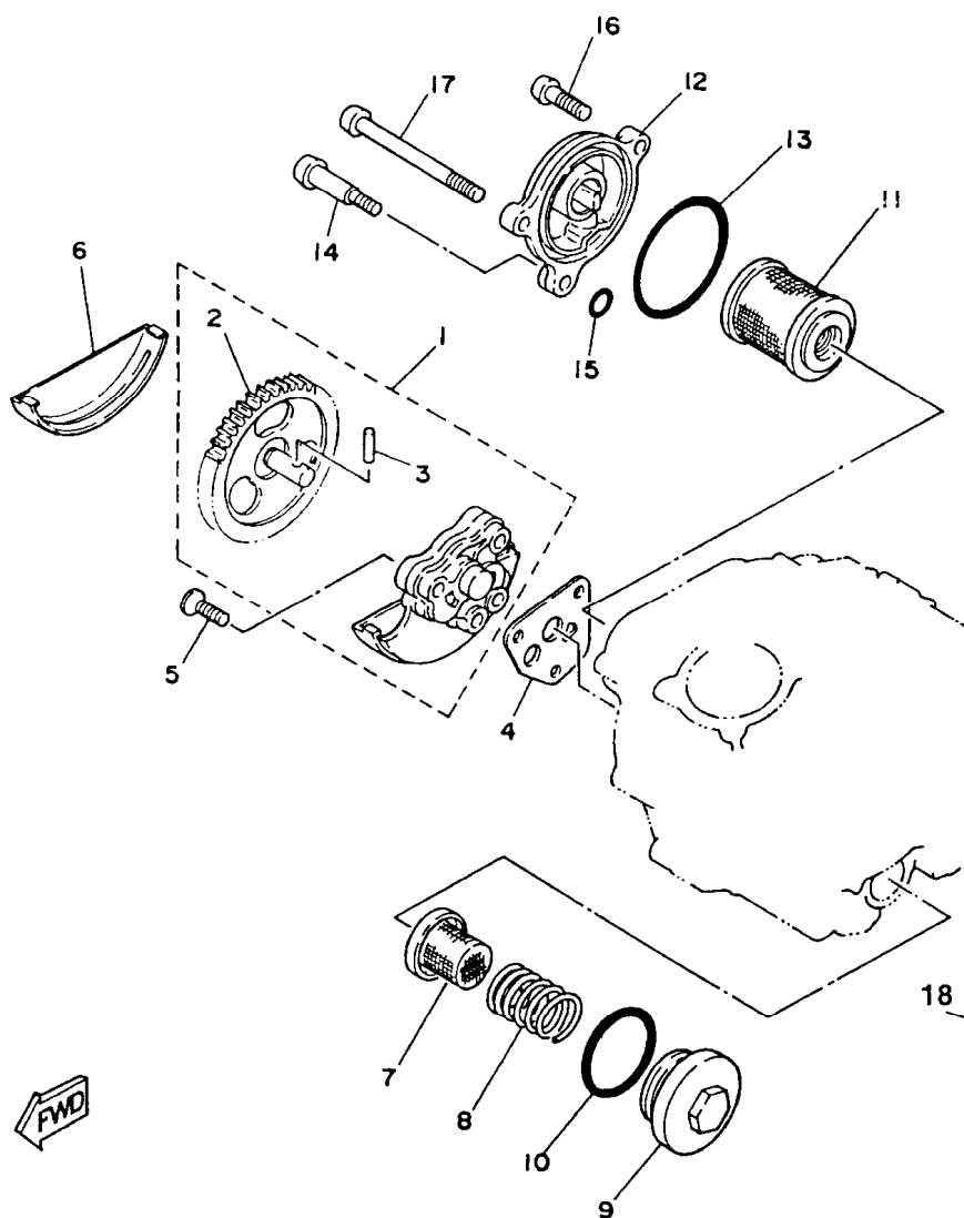
FIG. 06 - BOMBA DE ÓLEO
