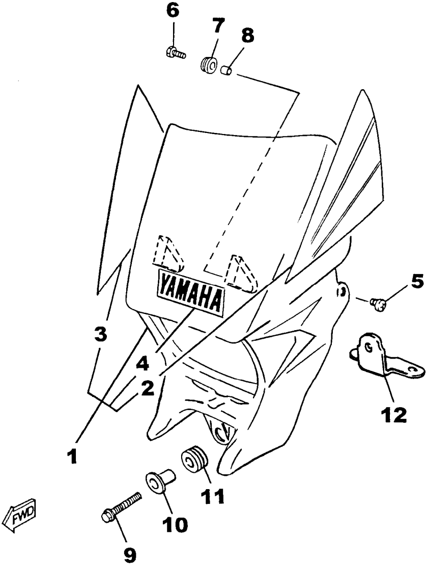
FIG. 28 - CARENAGEM
