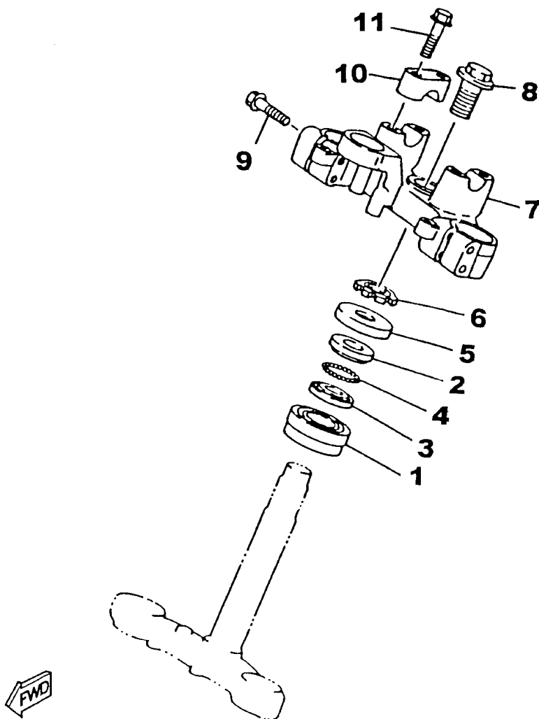
FIG. 21 - MESA DO GUIDÃO
