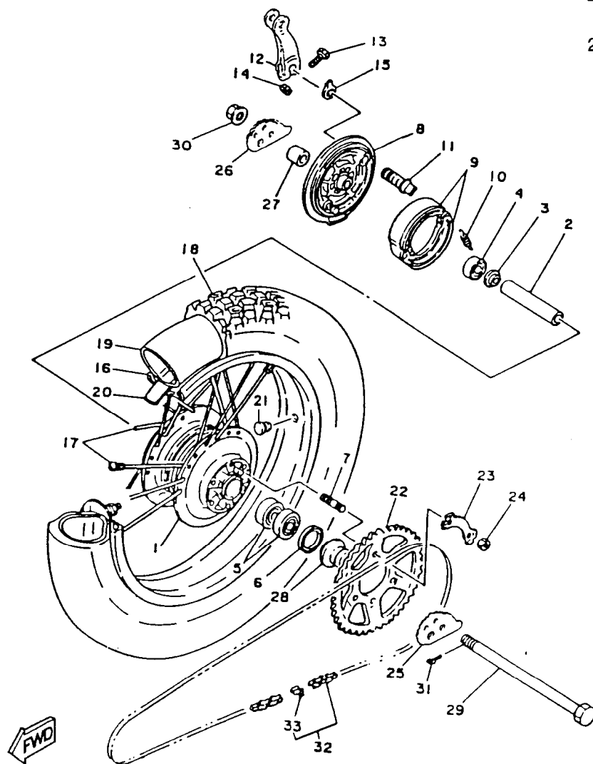
FIG. 24 - RODA TRASEIRA
