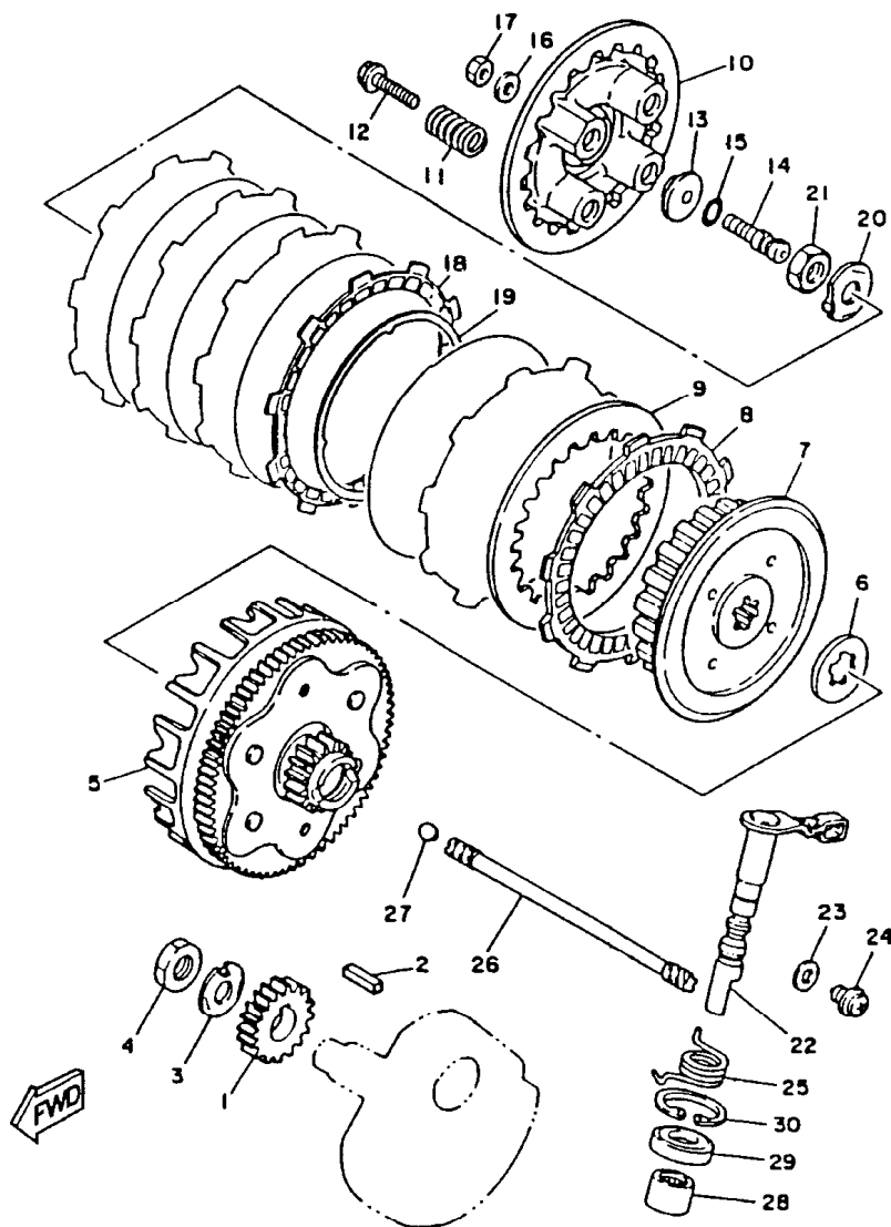
FIG. 12 - FRICÇÃO
