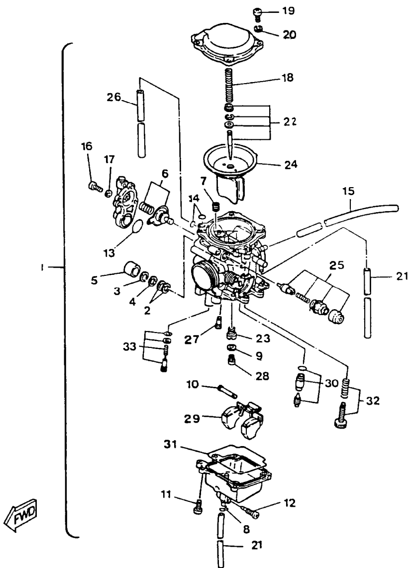
FIG. 16 - CARBURADOR
