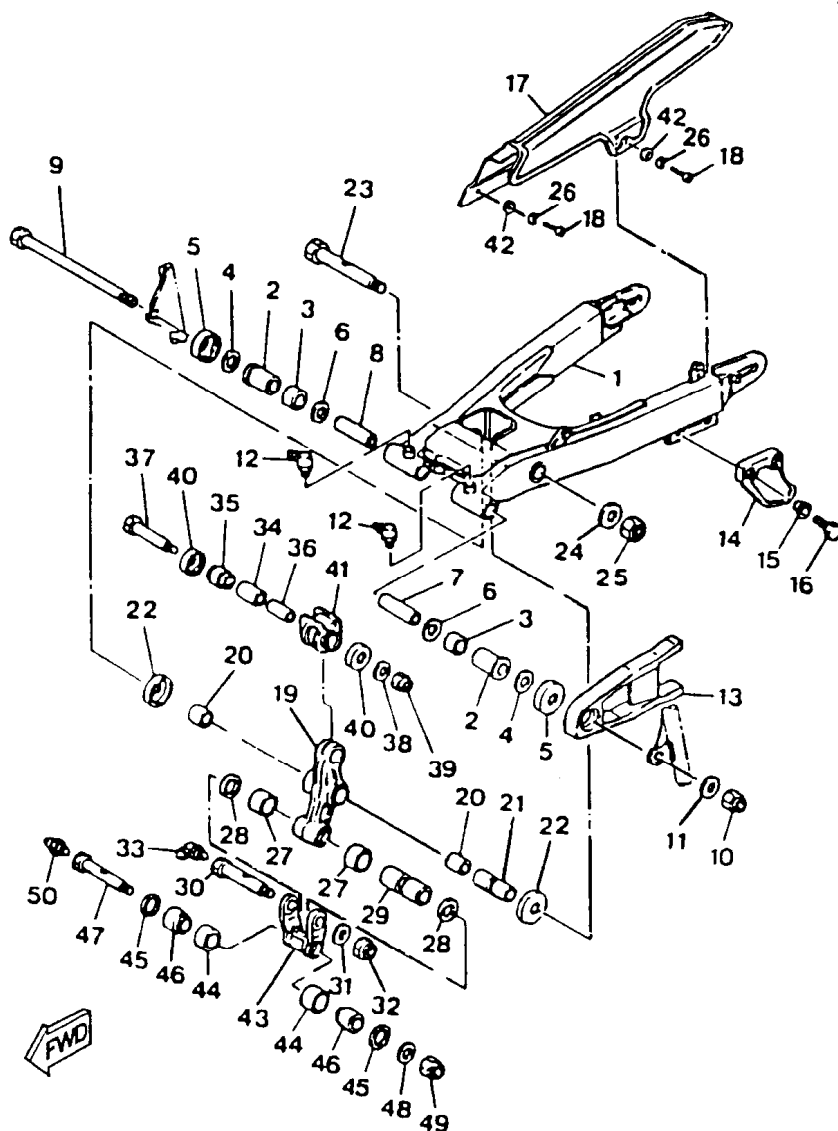
FIG. 19 - GARFO TRASEIRO
