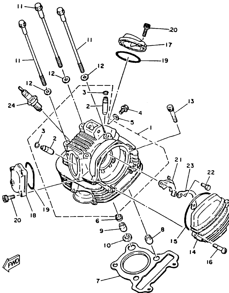
FIG. 01 - CABEÇOTE DO CILINDRO
