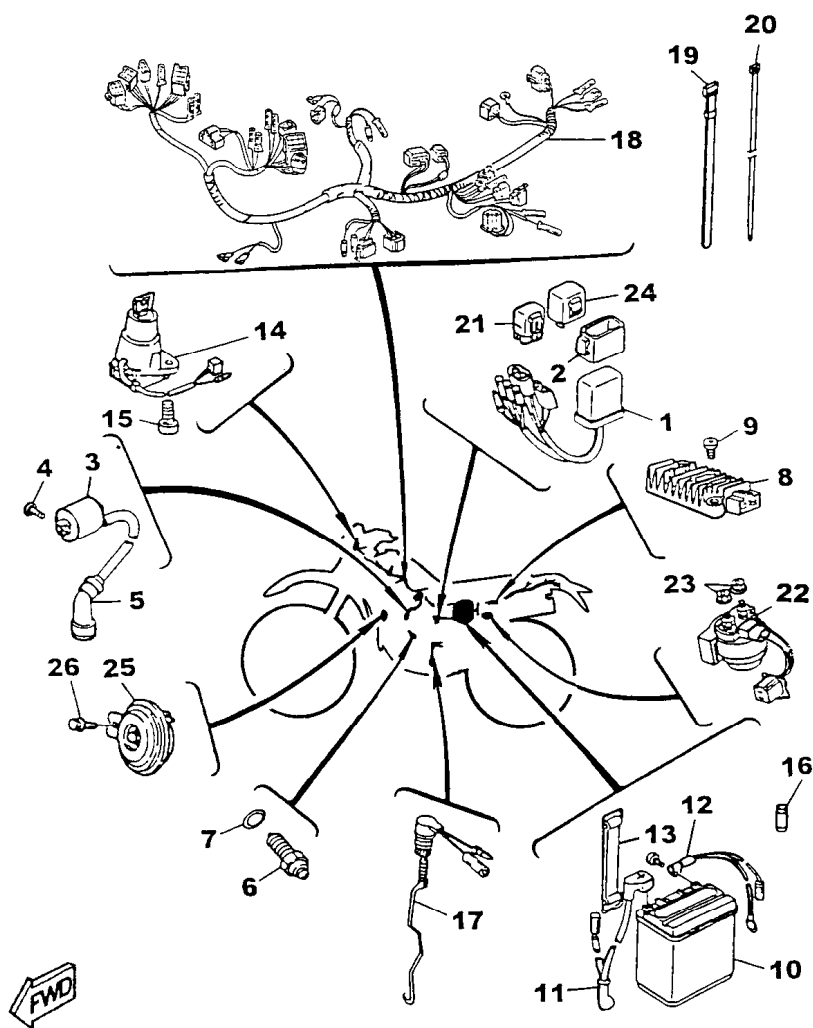
FIG. 41 - SISTEMA ELÉTRICO
