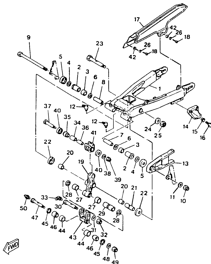
FIG. 19 - GARFO TRASEIRO
