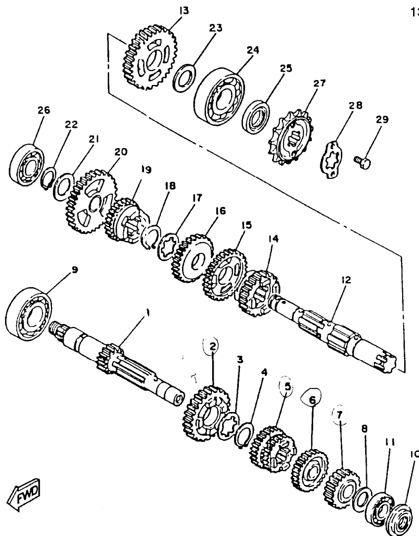
FIG. 13 - TRANSMISSÃO
