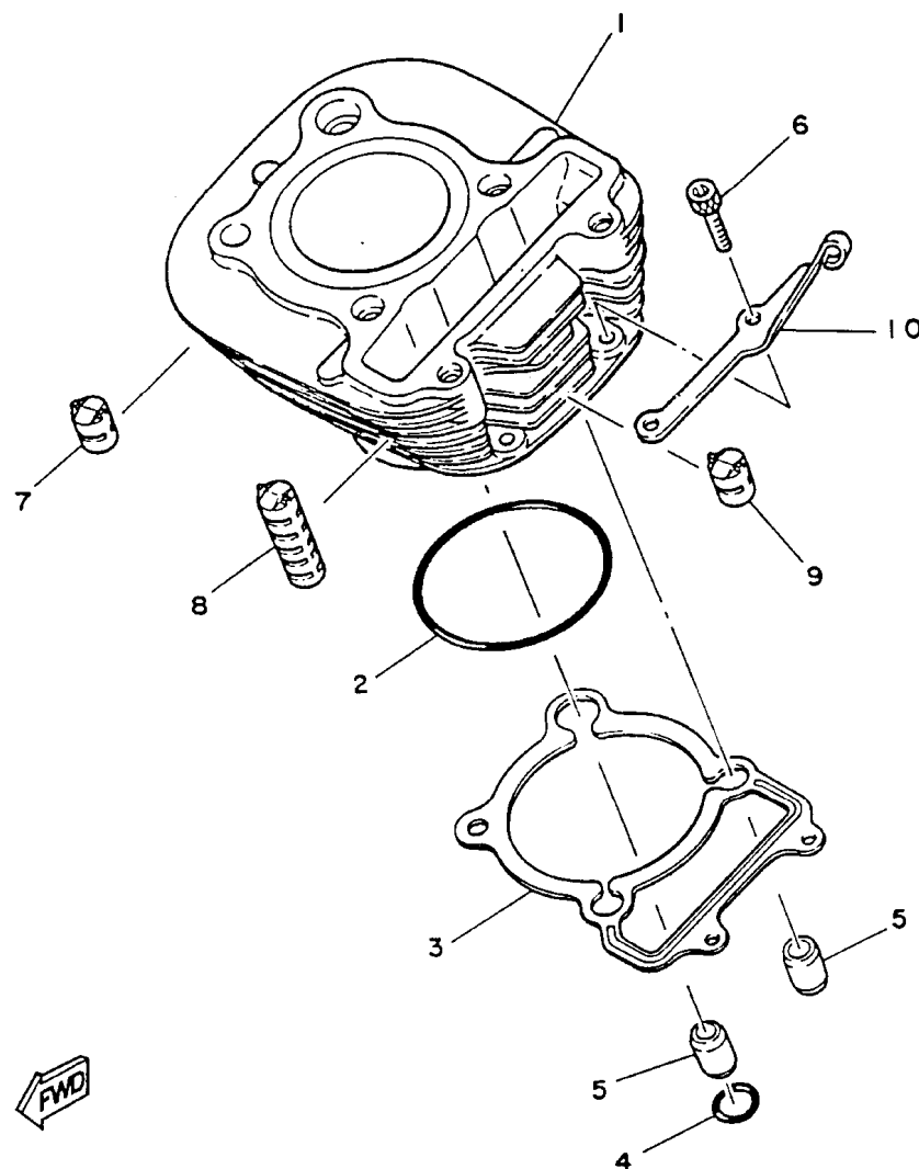
FIG. 02 - CILINDRO
