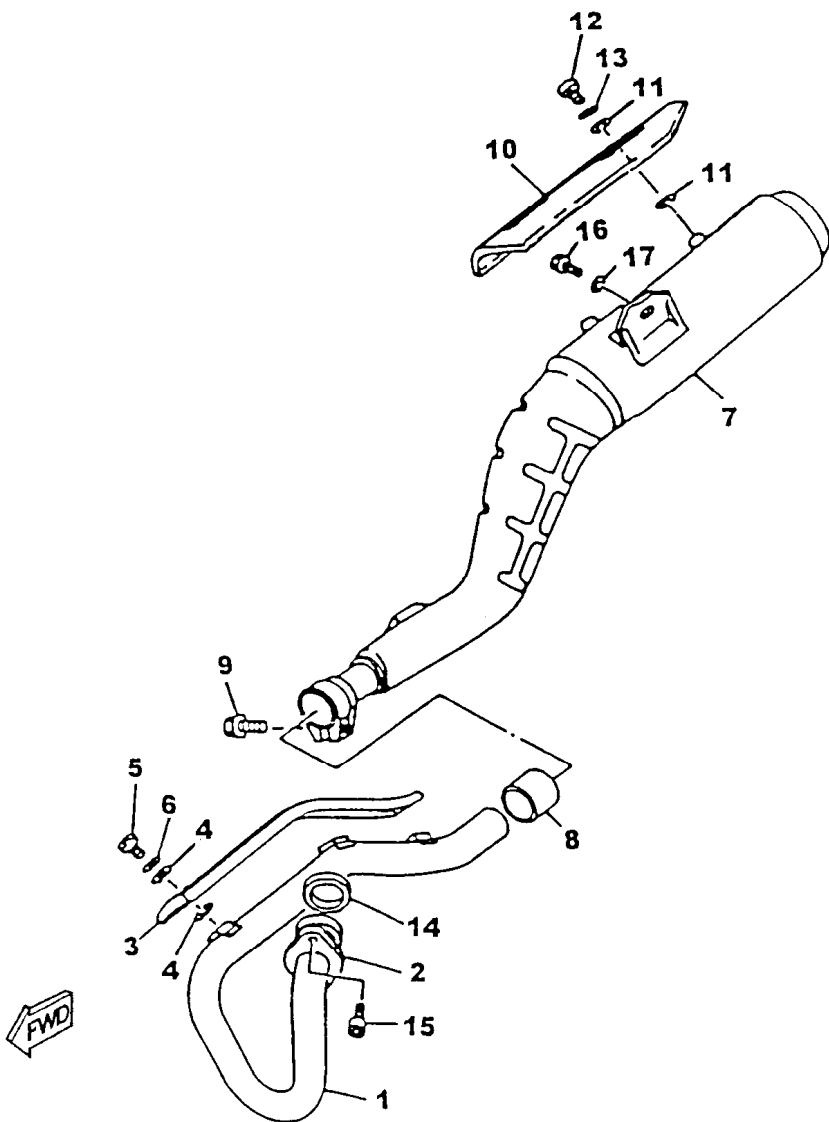
FIG. 08 - ESCAPAMENTO
