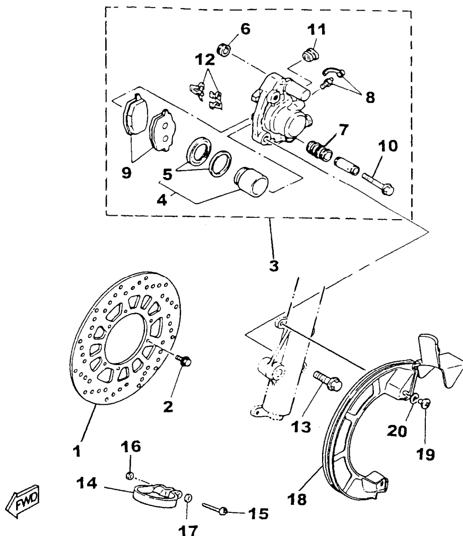
FIG. 23 - DISCO E PINÇA DO FREIO
