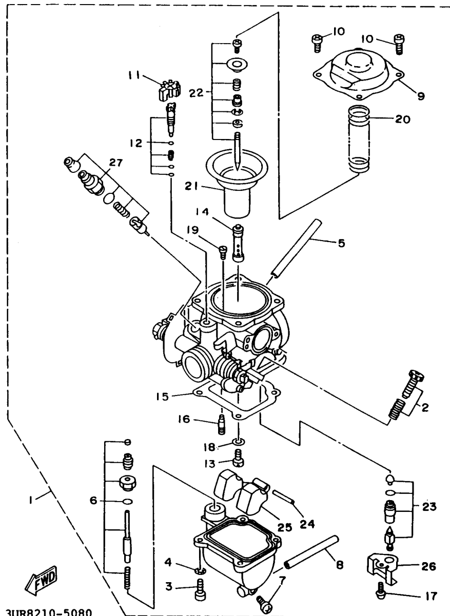
FIG. 8 CARBURETOR
