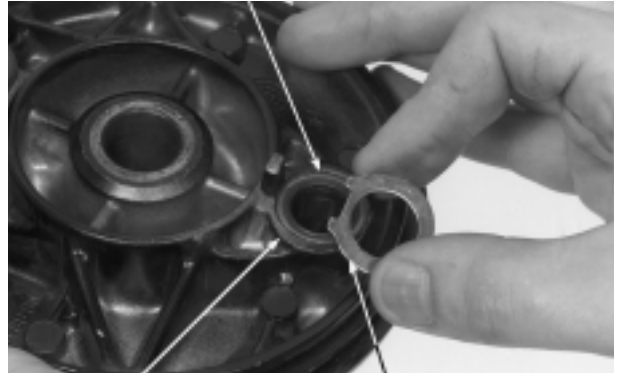
GRASA ASIENTO DE LA EXCENTRICA
