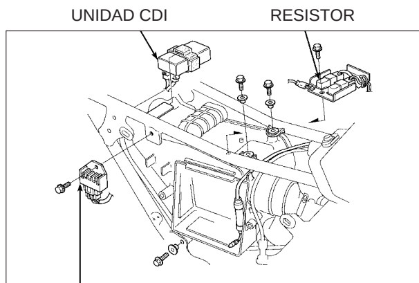
REGULADOR/RECTIFICADOR
