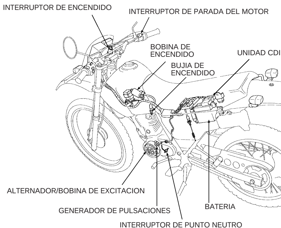
DIAGRAMA ELECTRICO:
