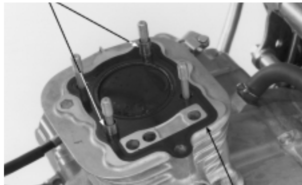
EMPAQUETADURA ARANDELA
