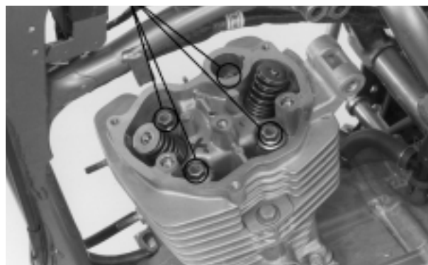
CULATA TORNILLOS
