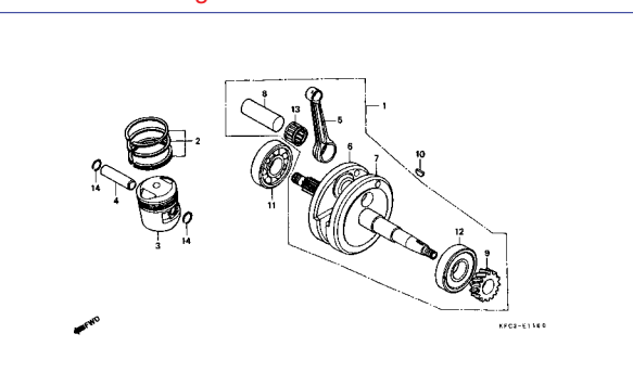
M-11 Árvore de Manivelas • Pistão / Crankshaft • Pistón / Cigüeñal • Pistón
