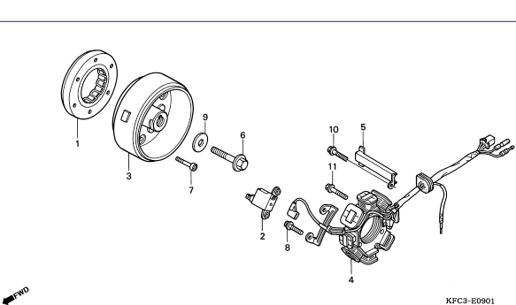
M-9.1 Gerador / Generator / Generator
