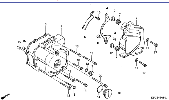
M-8.1 Tampa Lateral Esquerda / Left Crankcase Cover / Cubierta Izquierda del Cáster Motor
