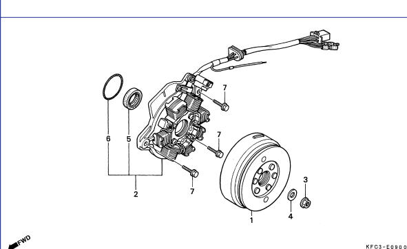
M-9 Gerador / Generator / Generator
