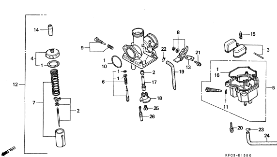
M-15 Carburador / Carburetor / Carburador
