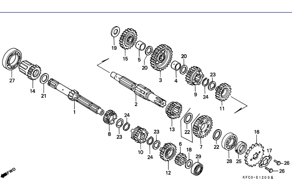
M-12 Transmissão / Transmission / Transmisión
