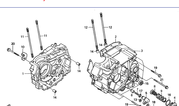
M-10 Carcaça / Crankcase / Cáster
