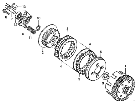
M-6 Embreagem / Clutch / Embrague
