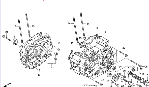
M-10.1 Carcaça / Crankcase / Cáster
