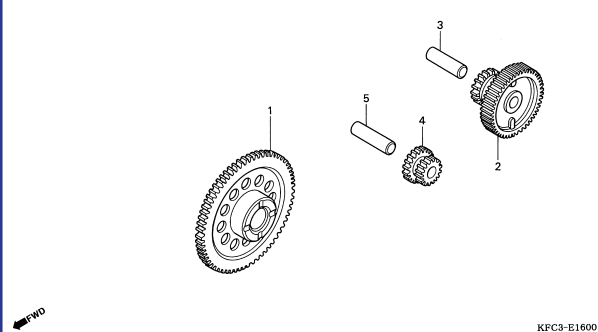
M-16 Engrenagem Partida / Starting Gear / Engranaje Arranque
