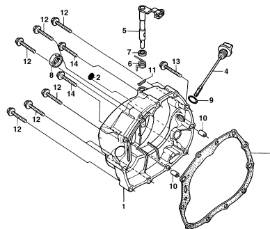
M-5 Tampa Lateral Direita / Right Crankcase Cover / Cubierta Derecha del Cáster Motor
