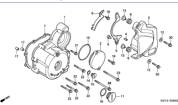
M-8.2 Tampa Lateral Esquerda / Left Crankcase Cover / Cubierta Izquierda del Cáster Motor
