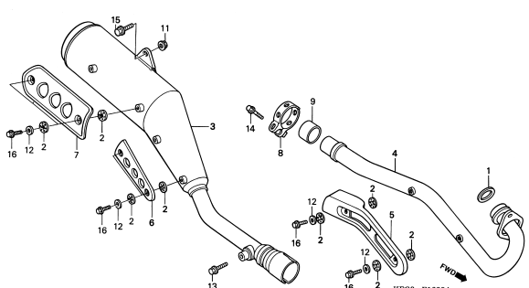
C-16 Escapamento / Exhaust Muffler / Silenciador de Escape
