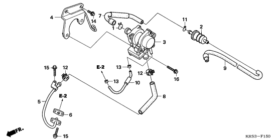
STEP
