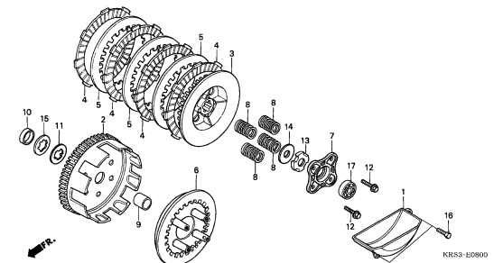
CLUTCH
