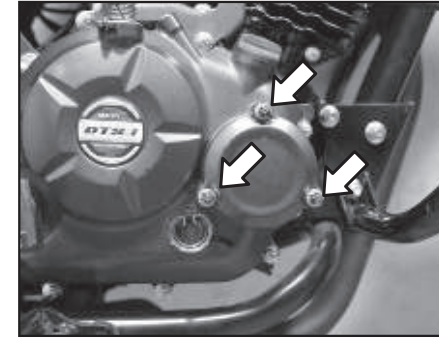
Tapa del filtro
