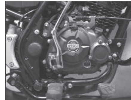
Pernos de la cubierta del embrague
