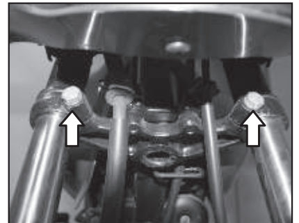
Pernos debajo del soporte del tenedor
