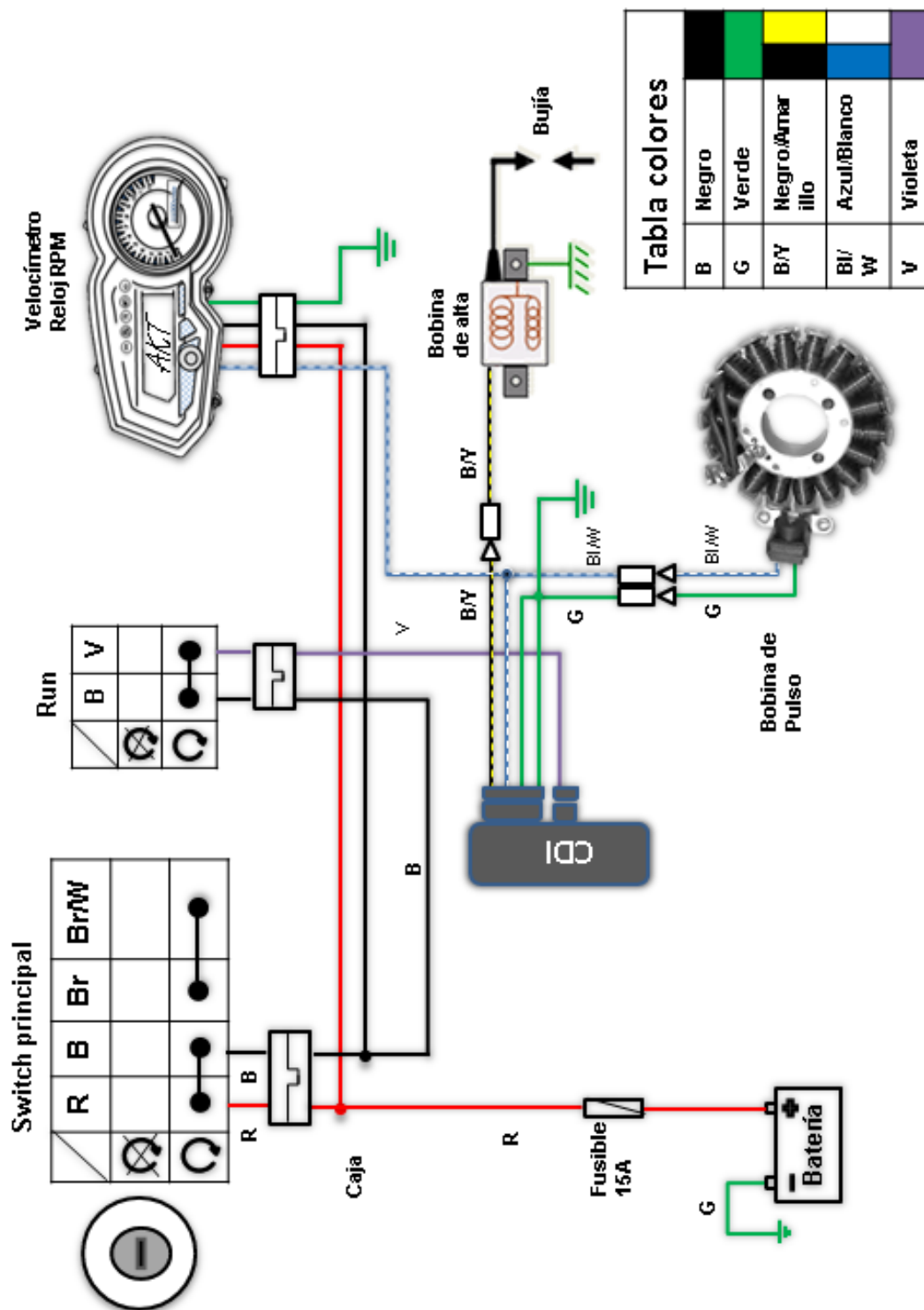
DIAGRAMA CIRCUITO DE ENCENDIDO RTX 150
